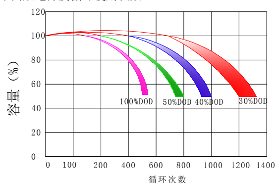
不同放电深度循环使用次数 (25°C)
