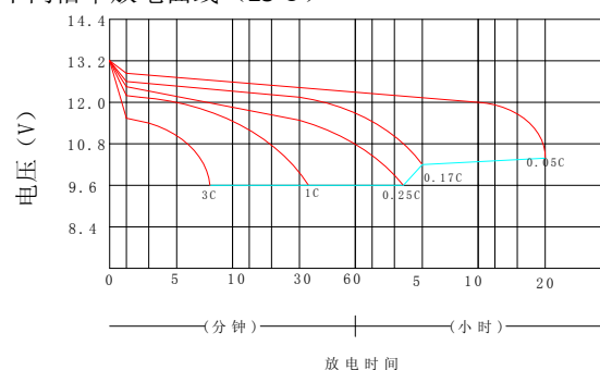
不同倍率放电曲线 (25°C)
