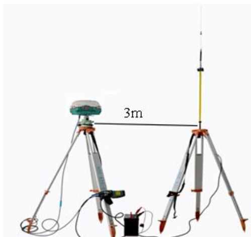
图 2-1 基准站的架设
