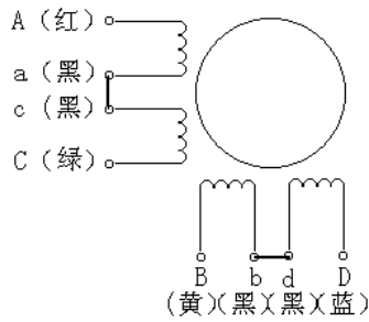
a) 串联接法
