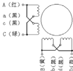
b) 并联接法
