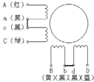
a) 串联接法
