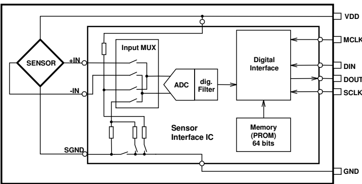
图1：MS5534C电路图
