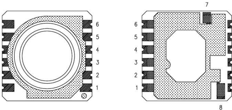
图2：MS5534C电气连接图
