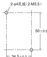
安装孔加工尺寸 (TOP VIEW)
