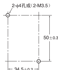
安装孔加工尺寸 (TOP VIEW)
