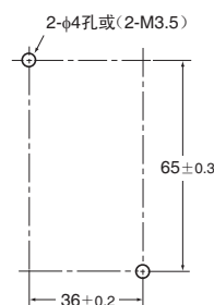
安装孔加工尺寸 (TOP VIEW)
