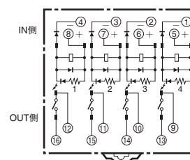
端子配置/内部连接图 (TOP VIEW)
